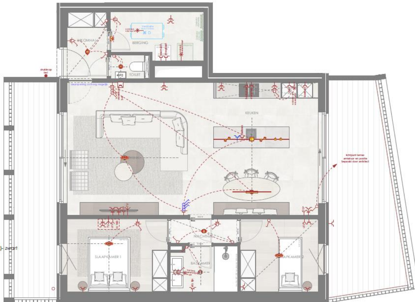
ELEKTRICITEITSPLAN APPARTEMENT 3.6
