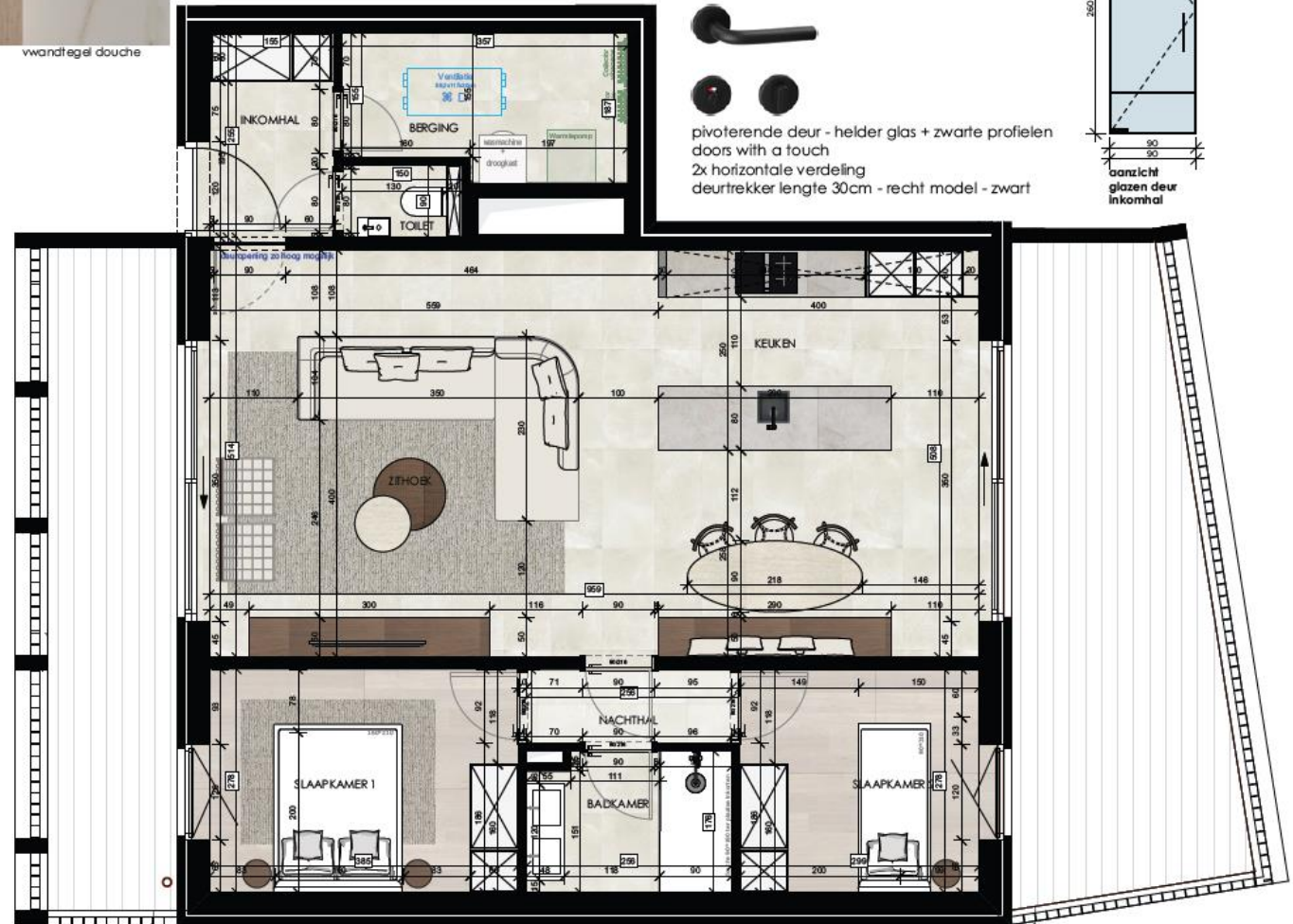
INTERIEURPLAN APPARTEMENT 3.6
